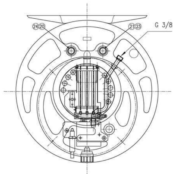
SEZ. A-A
