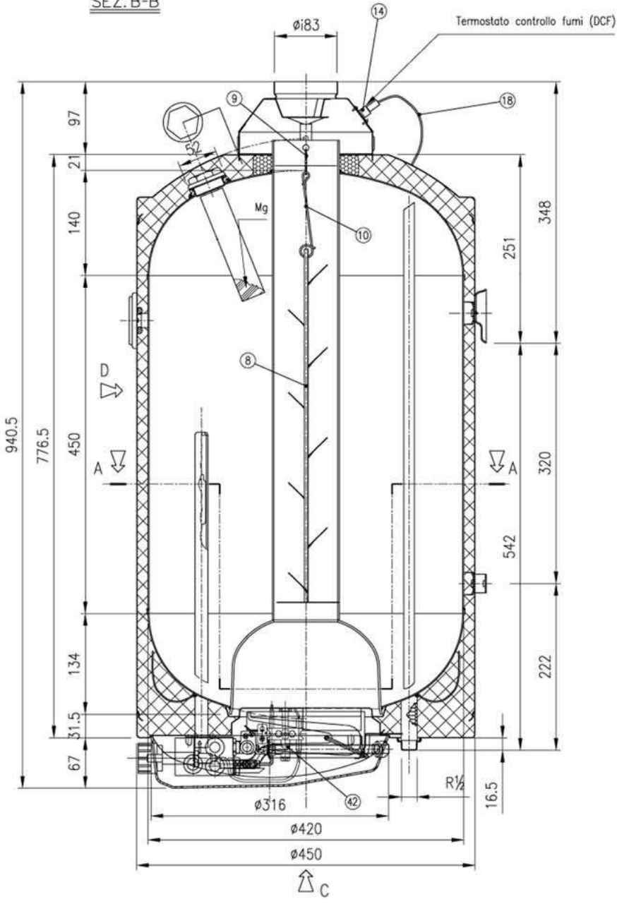
SEZ. B-B
