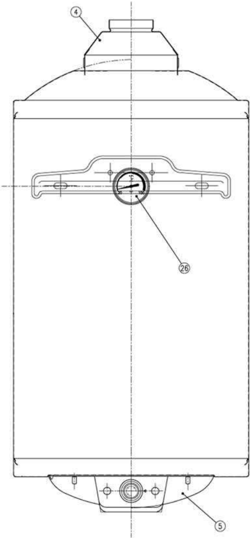
VISTA D
