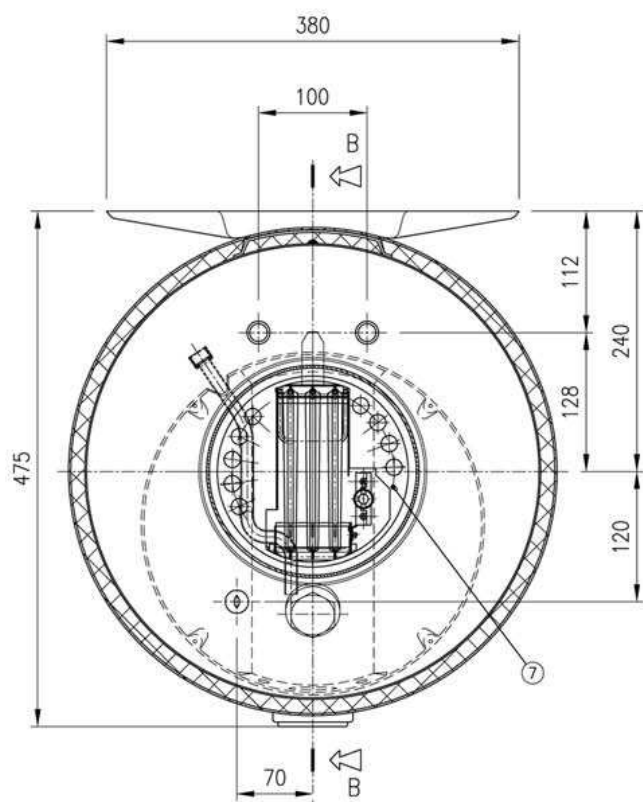
SEZ. A-A
