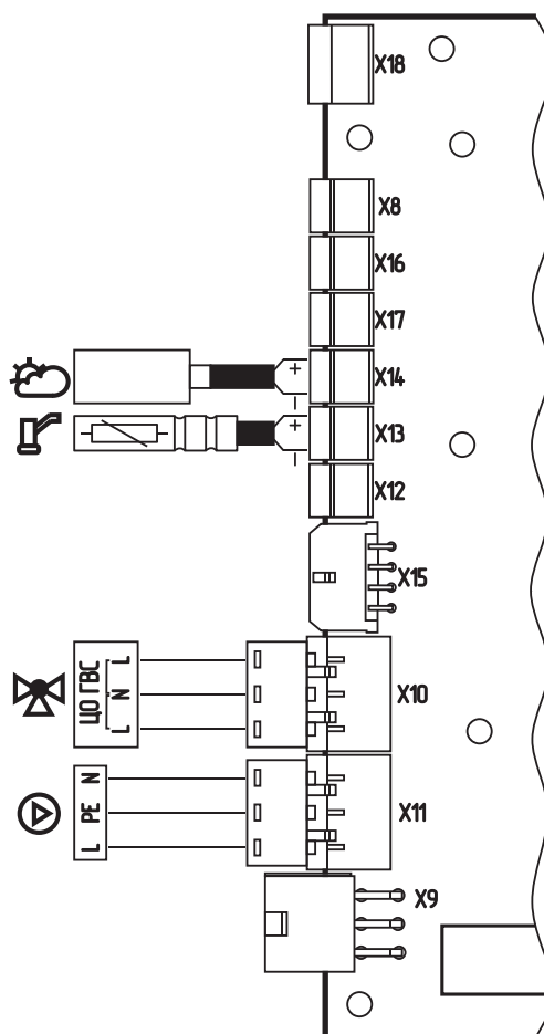
Рис.20 Подключение клапана приоритета бойлера ГВС, датчиков ГВС и улицы, к контроллеру «X-Line 100E»
