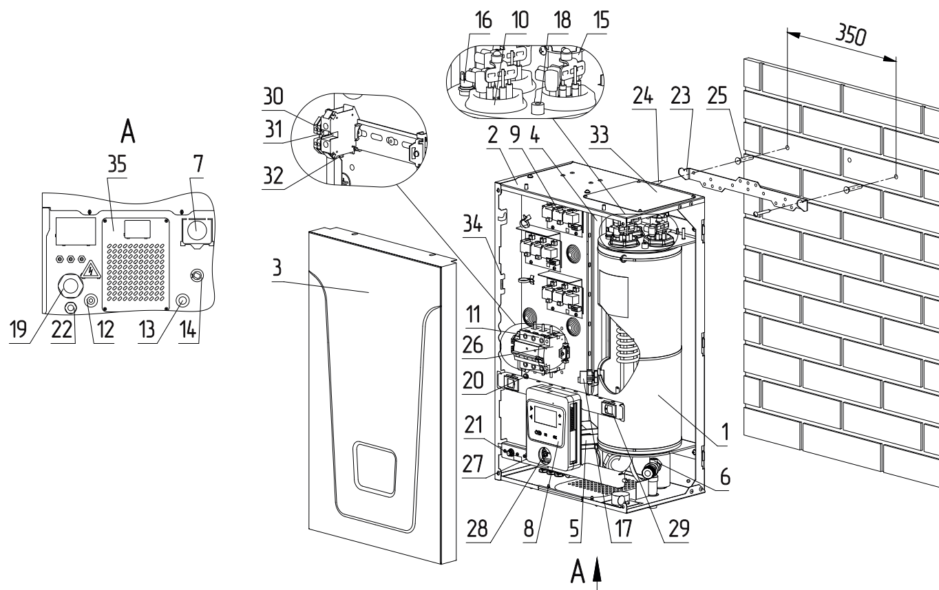
Рис.3 Конструкция котла
