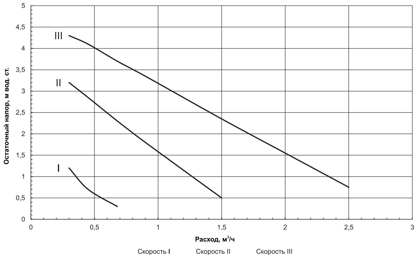
Рис.24 Напорные характеристики циркуляционного насоса 25/60 котлов BAXI AMPERA Plus 6-24 кВт
