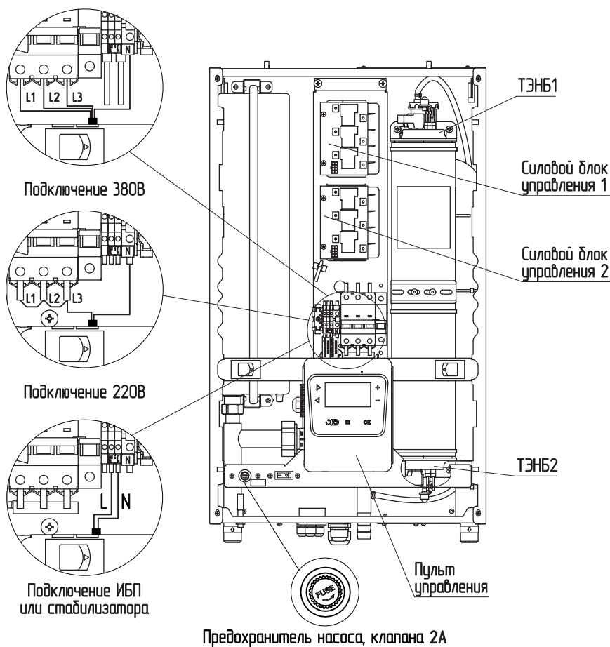
Рис.14 Органы управления электрического котла BAXI Ampere Plus 9-24 кВт
