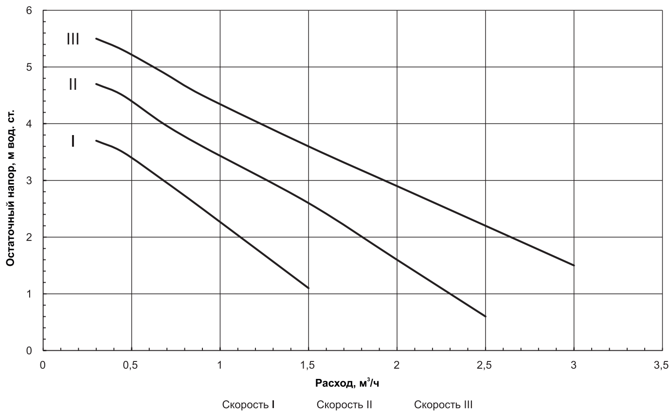
Рис.24.1 Напорные характеристики циркуляционного насоса 25/70 котлов BAXI AMPERA Plus 30-36 кВт
