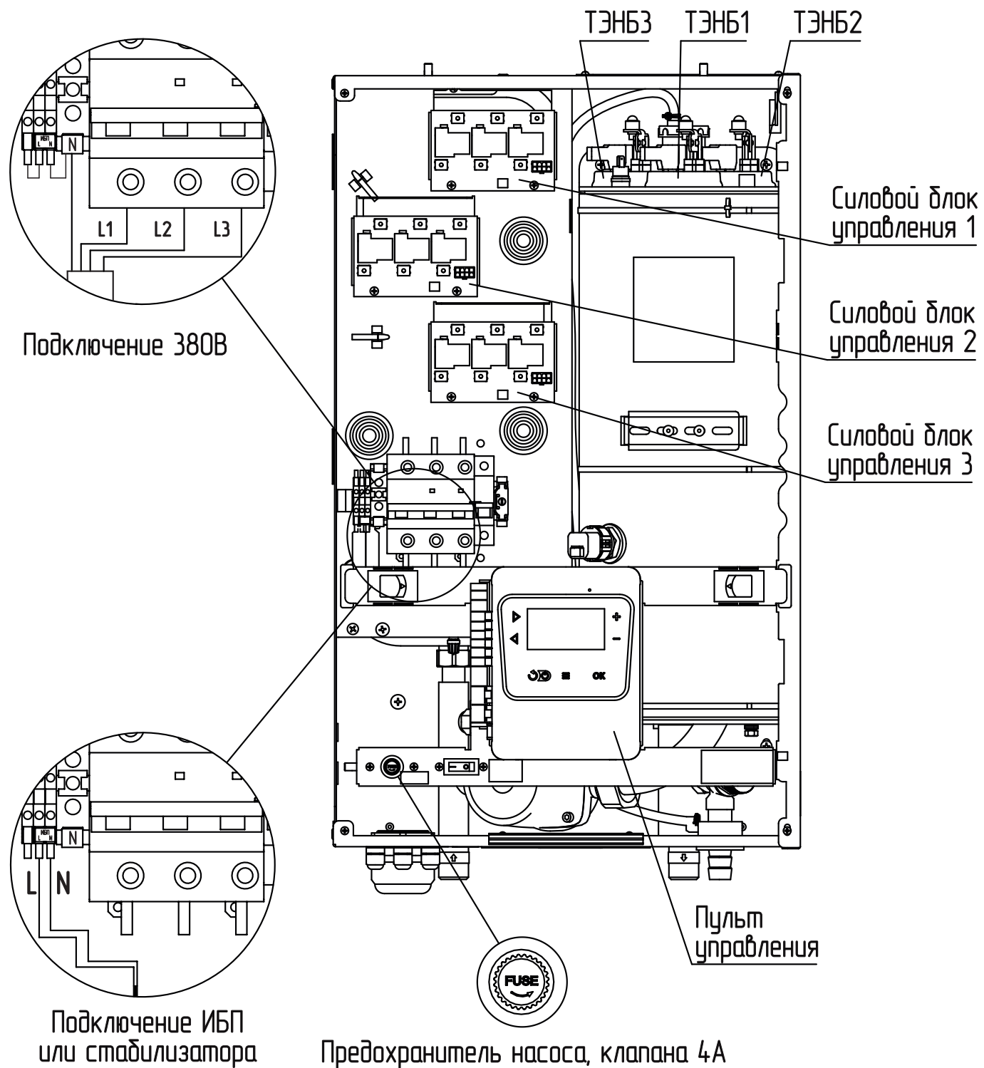
Рис.15 Органы управления электрического котла BAXI Ampere Plus 30-36 кВт
