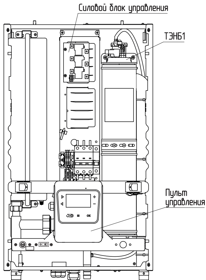
Рис.13 Органы управления электрического котла BAXI Ampere Plus 6 кВт
