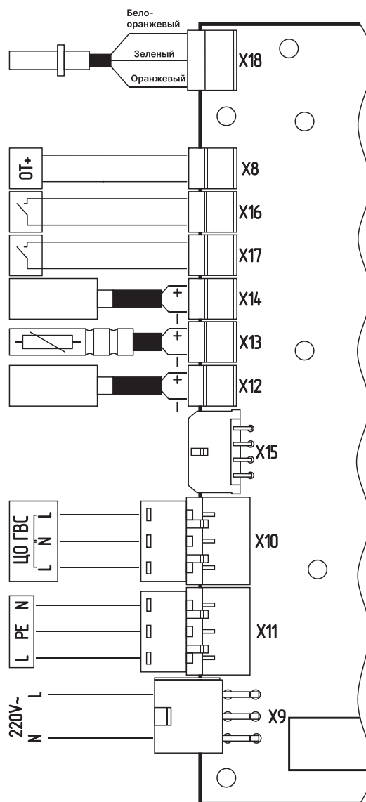
Рис.11 Схема подключения датчиков «X-Line100E»
