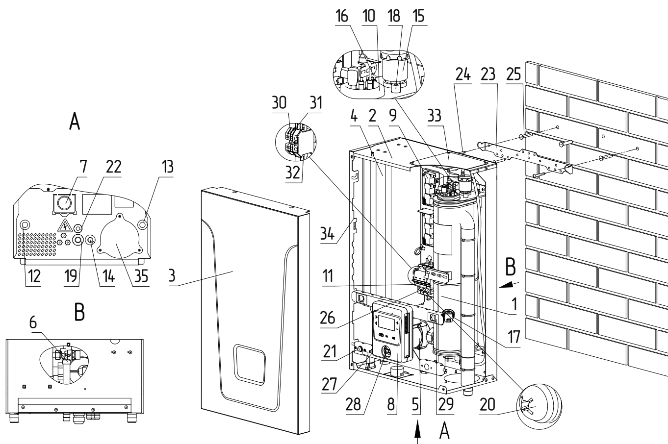
Рис.2 Конструкция котла
