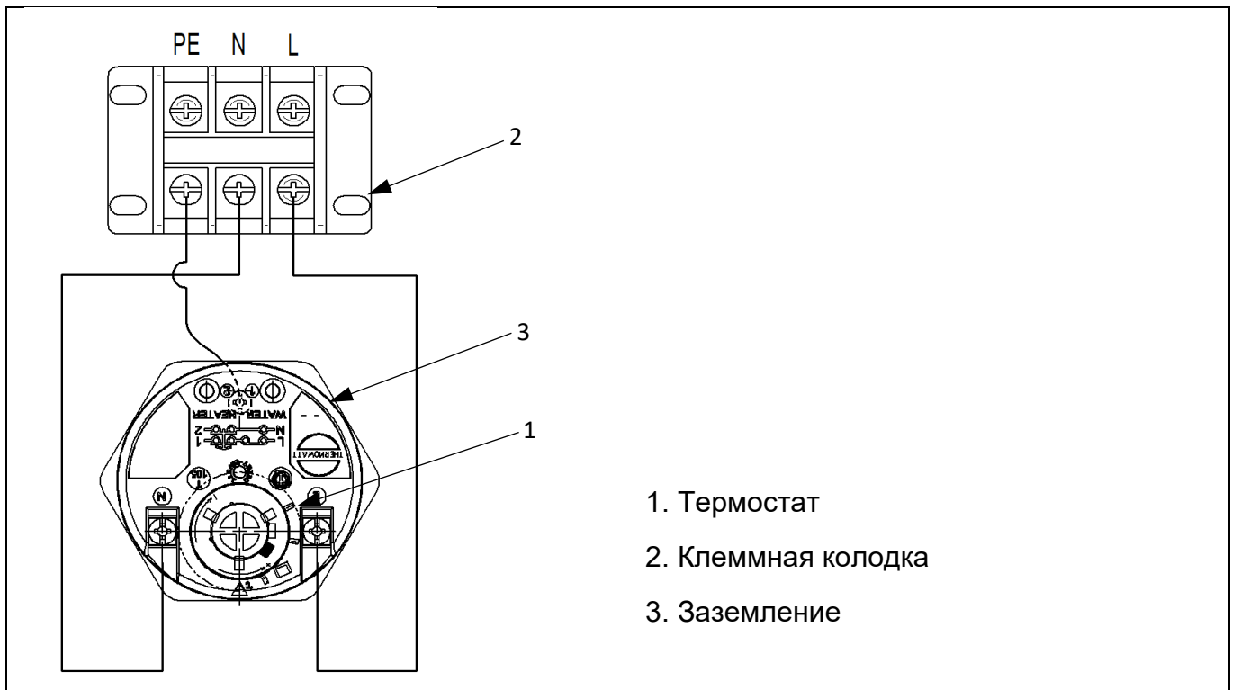
Рис. 3. Электрические элементы водонагревателя
