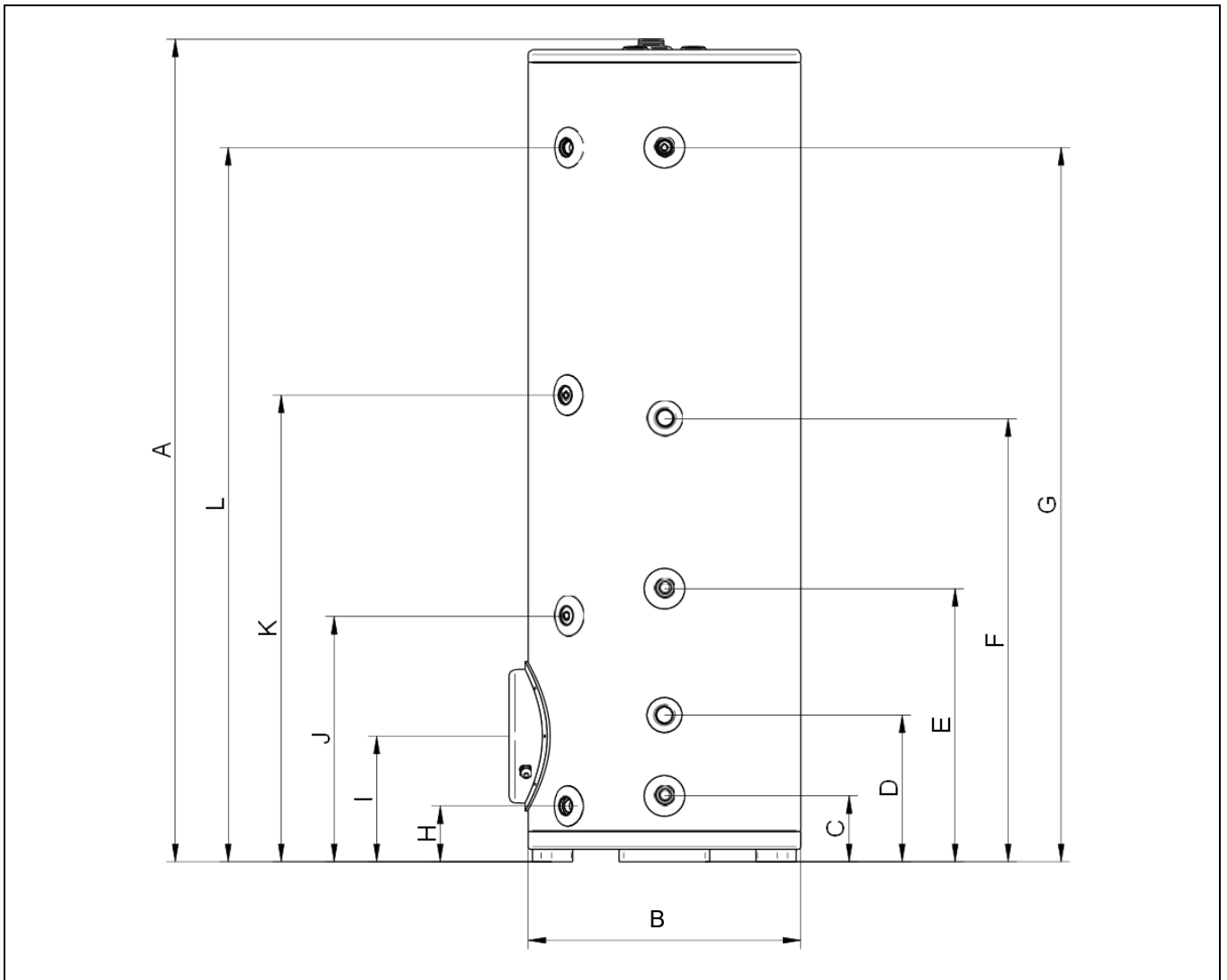
Рис. 2. Габаритные размеры водонагревателей UBC 150 Pro, 200 Pro, 300 Pro, 400 Pro, 500 Pro
