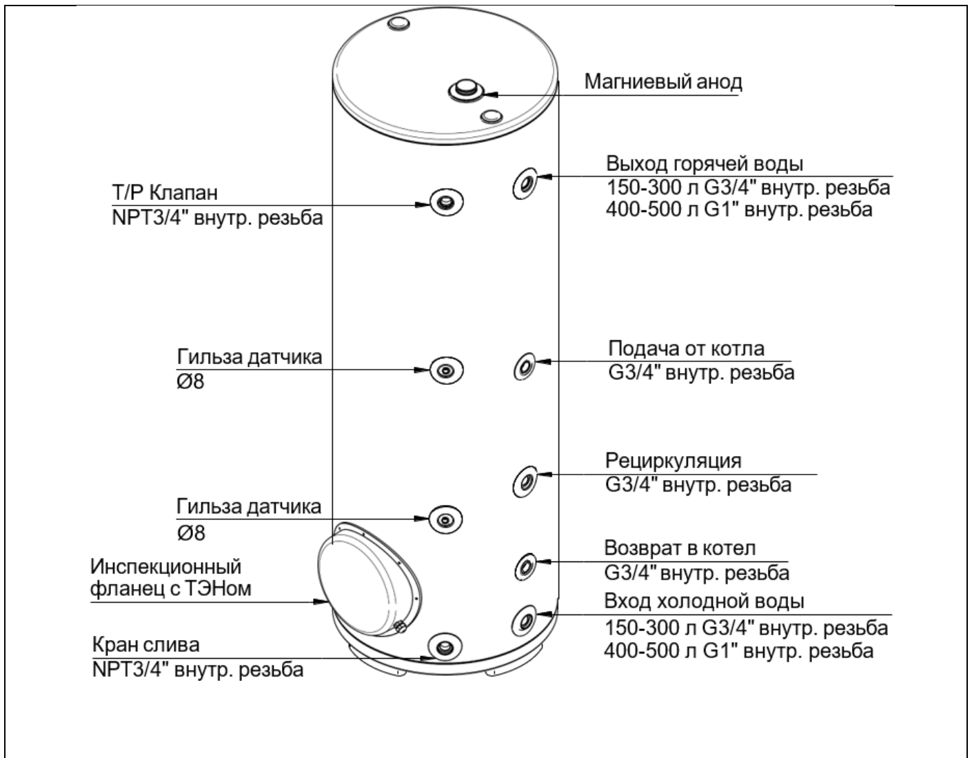
Рис. 1. Водонагреватель UBC 150 Pro, 200 Pro, 300 Pro, 400 Pro, 500 Pro
