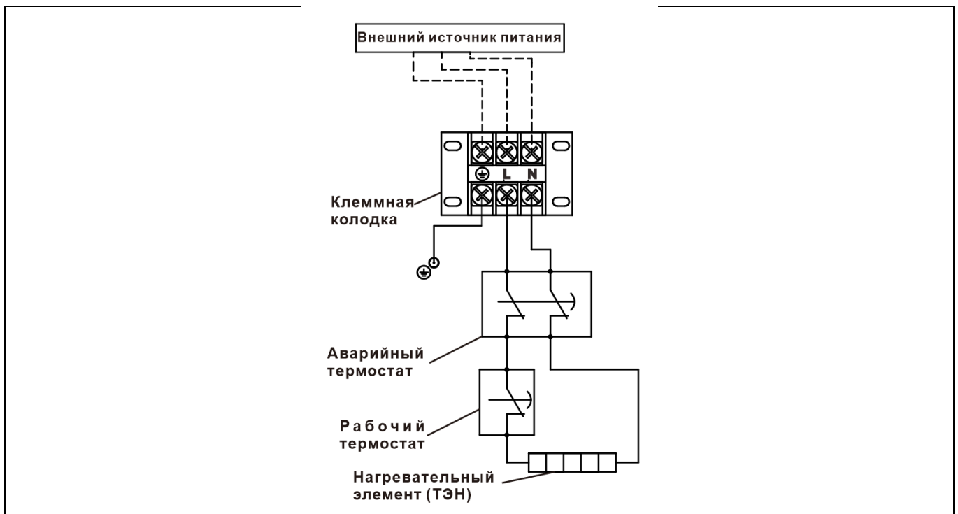
Рис. 4. Принципиальная электрическая схема и схема проводных подключений
